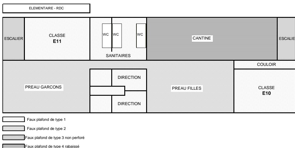
Figure 5 : Plan vu de dessus de l'école élémentaire du groupe scolaire des Bourdenières (rez-de-chaussée)
