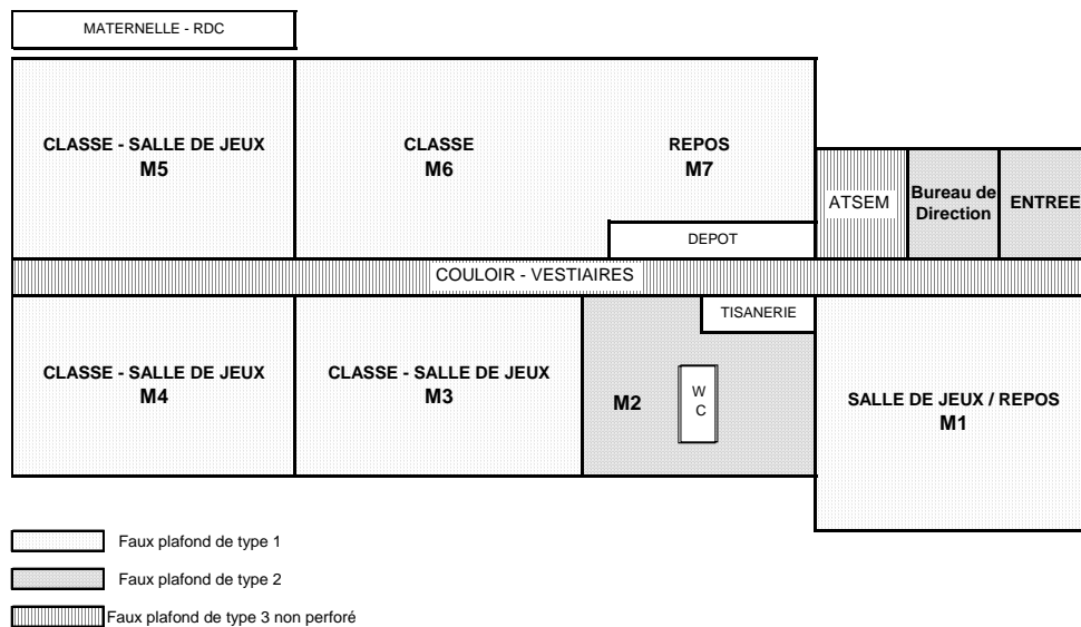
Figure 4 : Plan vu de dessus de l'école maternelle du groupe scolaire des Bourdenières (les types 1, 2 et 3 servant à différencier trois types de faux plafonds)
