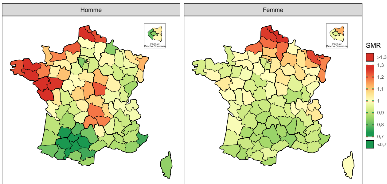
(c) Mortalité lissée 2007-2014, départements de France métropolitaine
