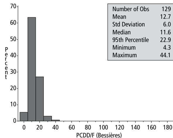
PCDD/F (Bessières)
