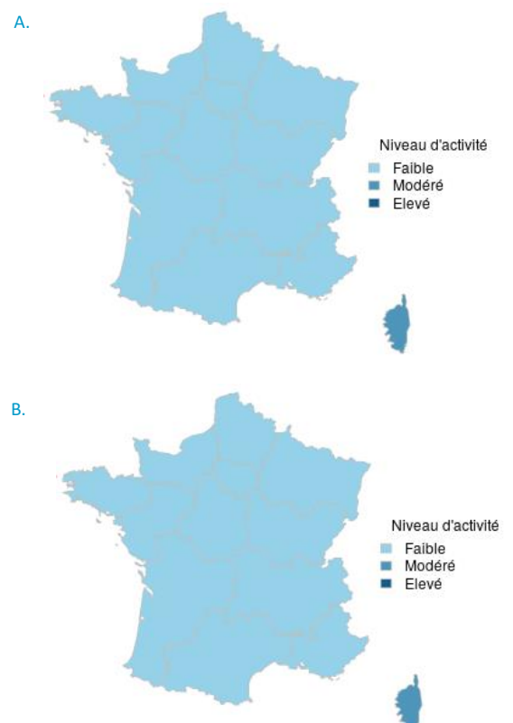
Figure 3 : Niveaux d'activité* pour GEA par région en semaine 47-2023, données SOS Médecins, France hexagonale (A) tous âges (B) moins de cinq ans
