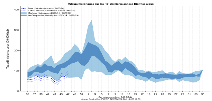
Figure 1: Taux d'incidence national (/ 100 000 habitants) de diarrhée aiguë, saisons 2012-2023, données du réseau Sentinelles au 28 novembre 2023
