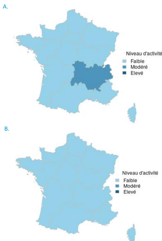
Figure 5: Niveaux d'activité* pour GEA par région en semaine 47-2023, données Oscour, France hexagonale (A) tous âges (B) moins de cinq ans
