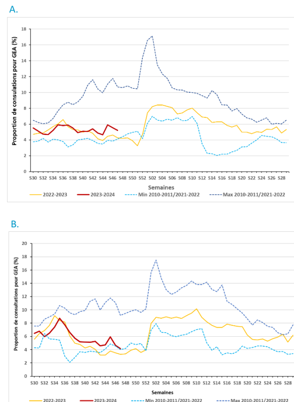
Figure 2: Proportion de consultations pour GEA, saisons 2022-2024, et minimums et maximums historiques (saison 2010-2011 à 2021-2022). Données SOS Médecins au 28 novembre 2023 (A) tous âges (B) moins de cinq ans
