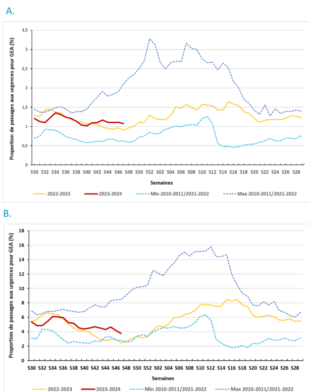
Figure 4: Proportion de passages aux urgences pour GEA, saisons 2022-2024, et minimums et maximums historiques (saison 2010-2011 à 2021-2022). Données Oscour au 28 novembre 2023 (A) tous âges (B) moins de cinq ans
