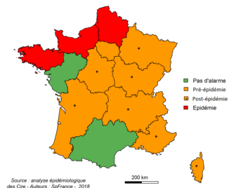
Figure 1– Niveau d'alerte régional pour les GEA en semaines 05/2018 et 06/2018, France métropolitaine
